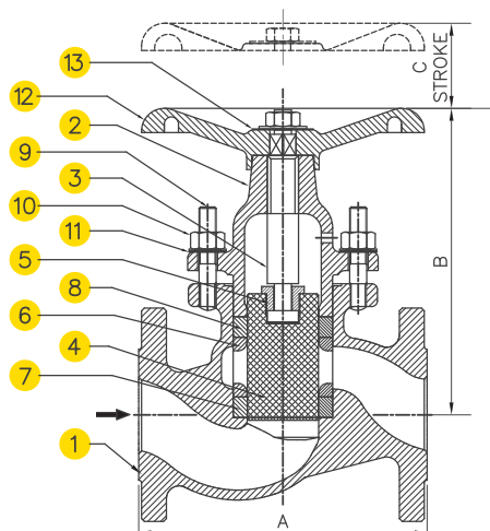
FIG. - DN15~DN50
